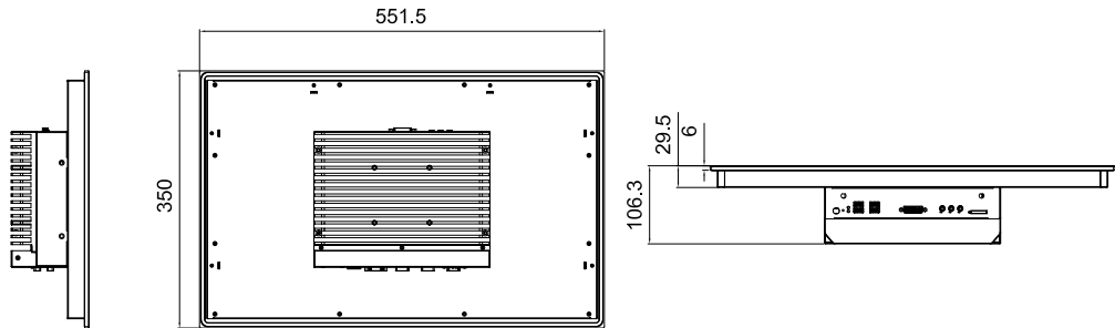
(具体配置尺寸, 见说明书) (单位:MM)
