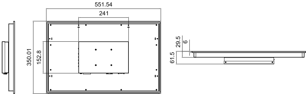
(具体配置尺寸, 见说明书) (单位:MM)
