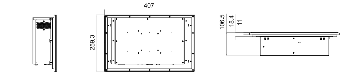
(具体配置尺寸, 见说明书) (单位:MM)
